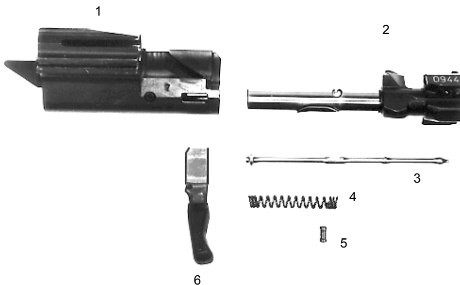
Bild 4: Verschluss zerlegt
