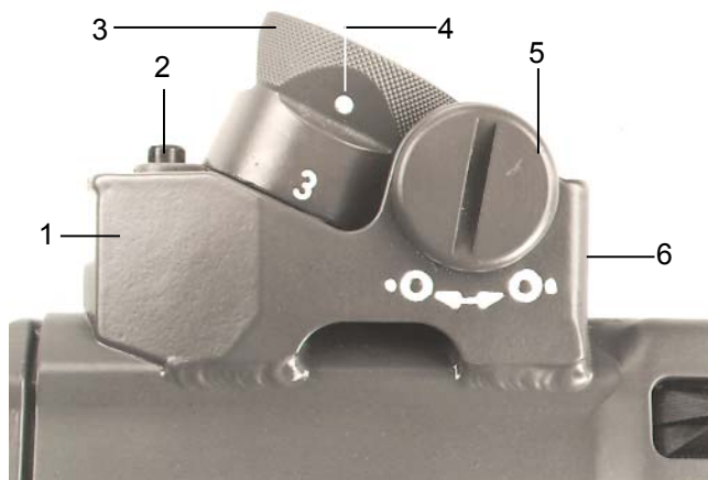
Bild 7: Diopter-Visier
