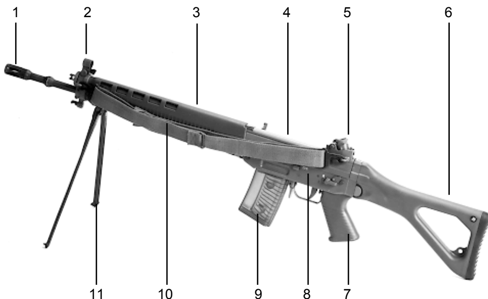
Bild 1: Bestandteile des 5,6 mm Stgw 90
